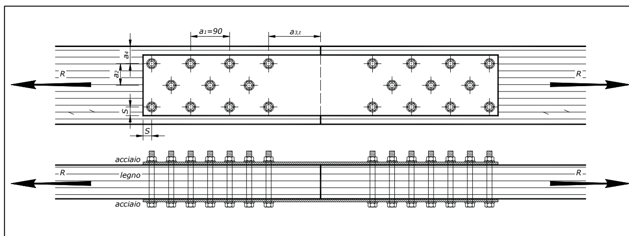
Figura 17-5 –Schema del collegamento
